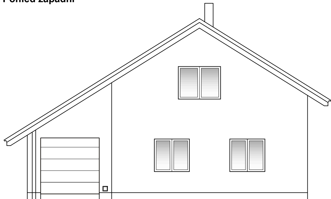
Pohled západní
