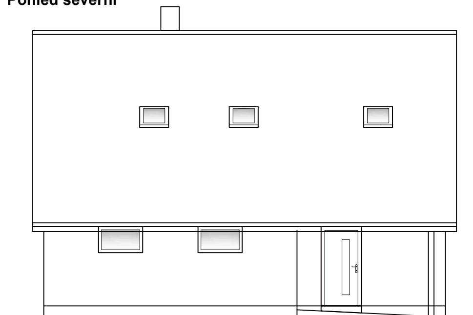
Pohled severní
