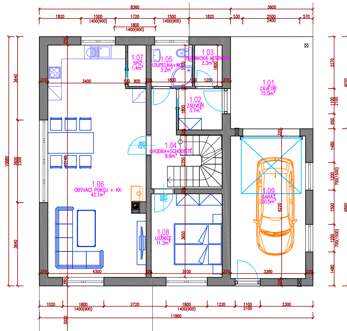
PŮDORYS 1.NP
