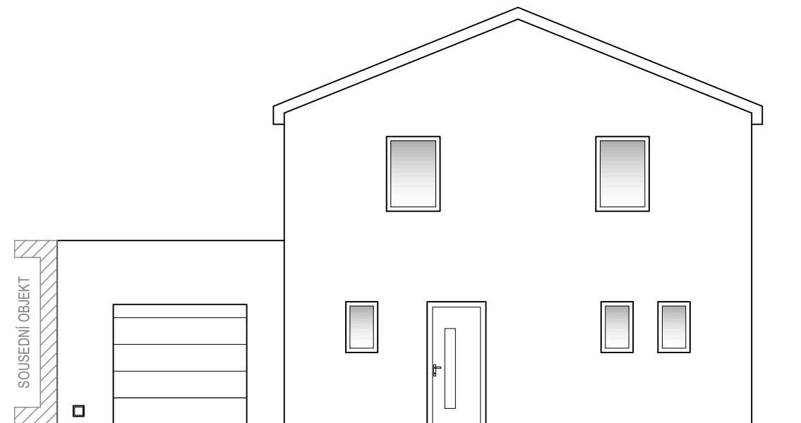
Pohled východní
